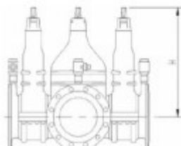
Schieber mit Servicehahn
